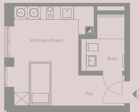
1. OBERGESCHOSS | WE 04
