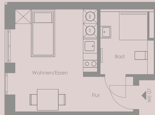
1. OBERGESCHOSS | WE 07
