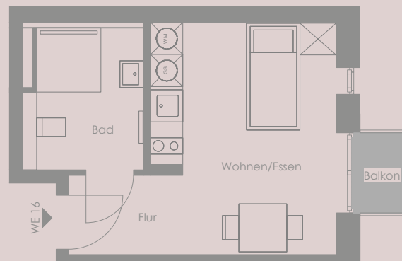
2. OBERGESCHOSS | WE 16
