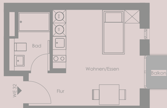
4. OBERGESCHOSS | WE 32
