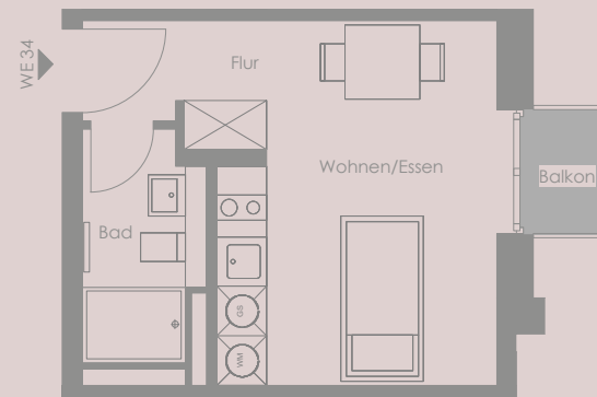
4. OBERGESCHOSS | WE 34
