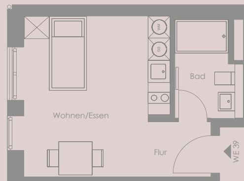
5. OBERGESCHOSS | WE 39
