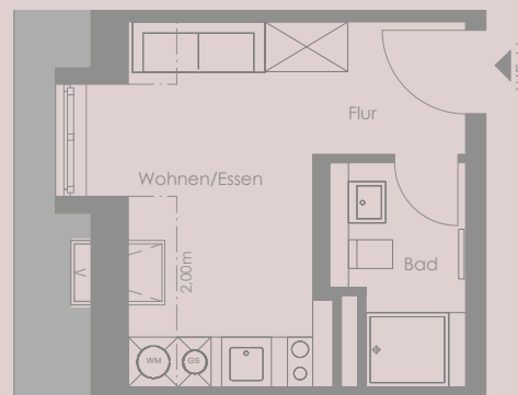
6. OBERGESCHOSS | WE 46
