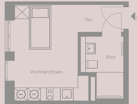
2. OBERGESCHOSS | WE 14
